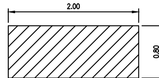
焊盘尺寸 尺寸公差 ±0.05
